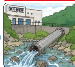
新川発電所付近の導水管が河川へ転落していることを確認
